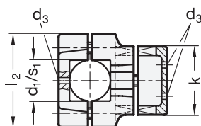
Śruba z łbem walcowym / Nakrętka sześciokątna
